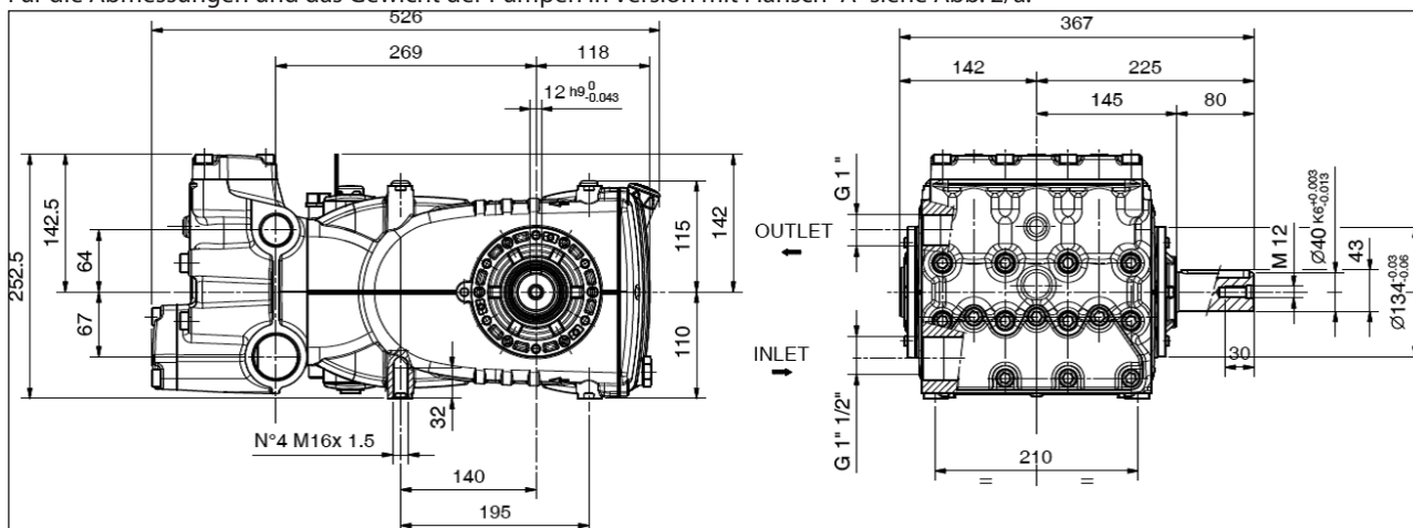
Trockengewicht 70 kg.
