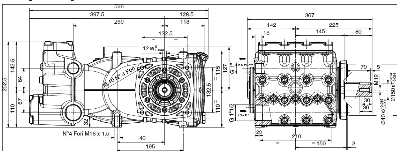
Trockengewicht 71 kg.
